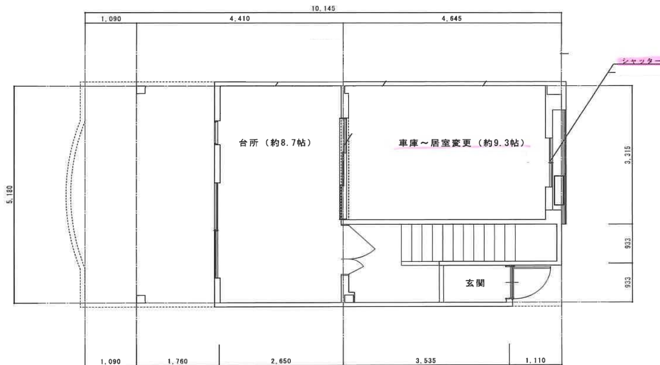
【 1 階平面図 S = 1/50 】
