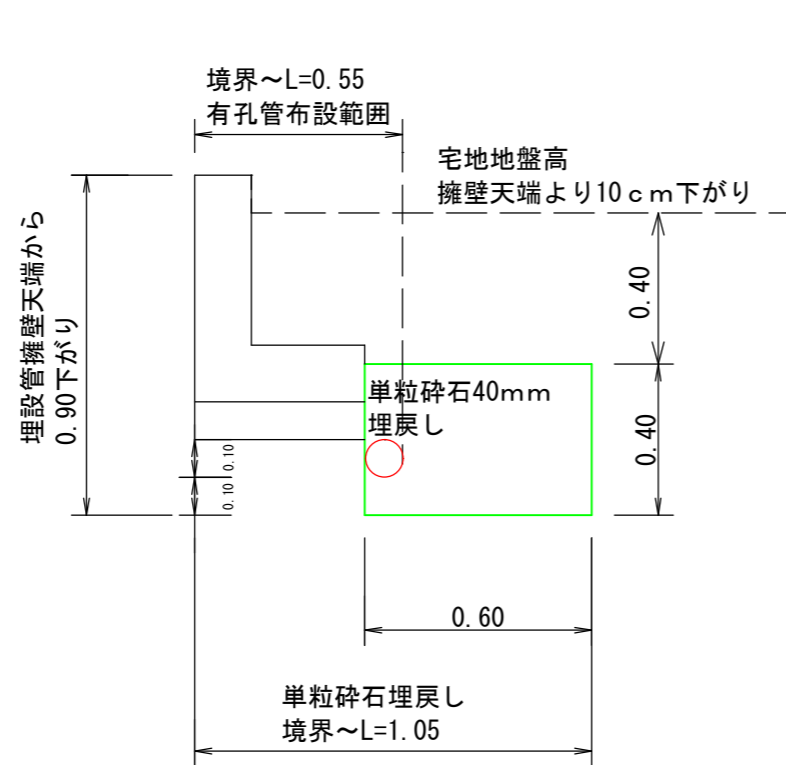
①号地構造図面
