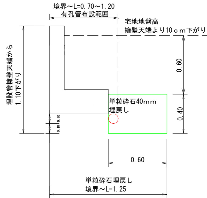
②号地構造図面
